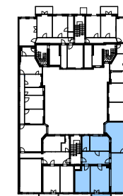
Geschossplan: 4. OG
